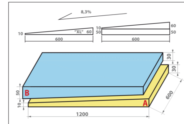
Рис. 3.3.11 Укладка ПВХ-мембраны в разуклонке из клиновидных плит
