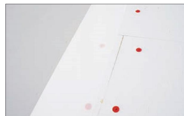
Рис. 3.2.1 Крепление мембраны и плит утепления с предварительным прокалыванием в случае использования жестких полимерных материалов (XPS, PIR)
