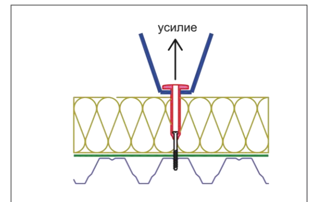
Рис. 3.5.8 Визуальный метод определения надежности установки крепежа
