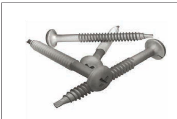
Рис. 4.5.2 Кровельный саморез остроконечный ТЕХНОНИКОЛЬ в сочетании с полиамидной гильзой
