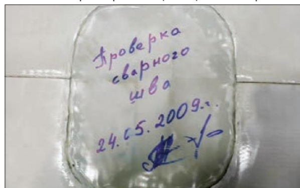
Рис. 5.2.12 Знак качества сварного шва
