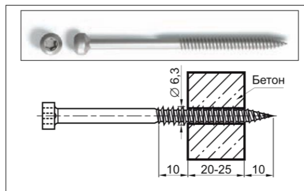
Рис. 2.10.1 Саморез по бетону 06,3 мм
