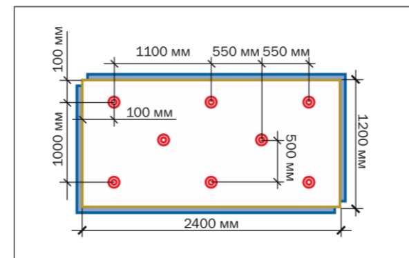
Рис. 2.2.4 Рекомендуемая схема крепления плит теплоизоляционных PIR
