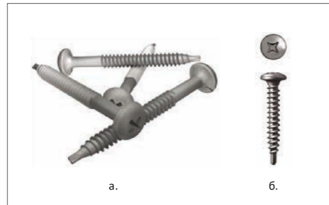
Рис. 3.5.11 Кровельный саморез сверлоконечный ТЕХНОНИКОЛЬ. а. \varnothing 4,8; б. \varnothing 5,5
