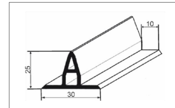
Рис. 4.8.1 Профиль для имитации стоячего фальца
