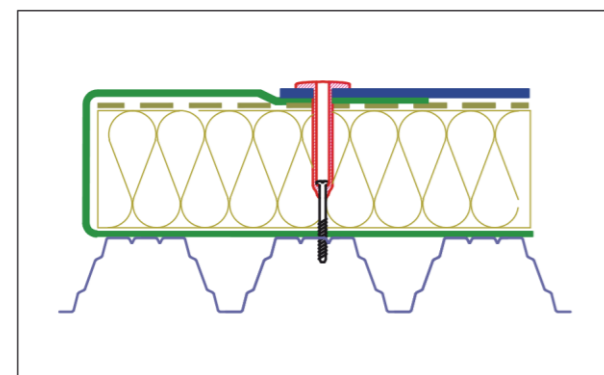
Рис. 3.1.6 Защита теплоизоляции от намокания
