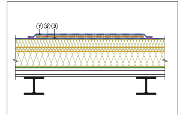
1. Готовый элемент LOGICROOF WalkWay Puzzle.
