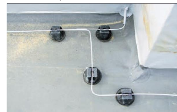
Рис. 4.8.14 Молниезащита ТЕХНОНИКОЛЬ
