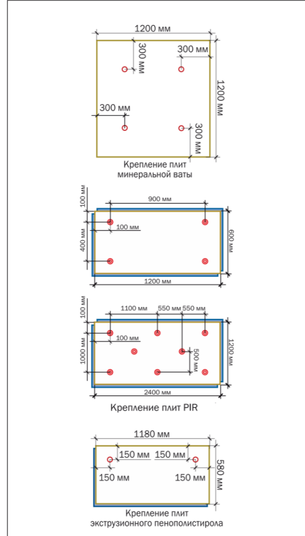
Рис. 3.5.4 б Крепление плитной теплоизоляции многослойного утепления нет необходимости крепить каждый слой отдельно.
