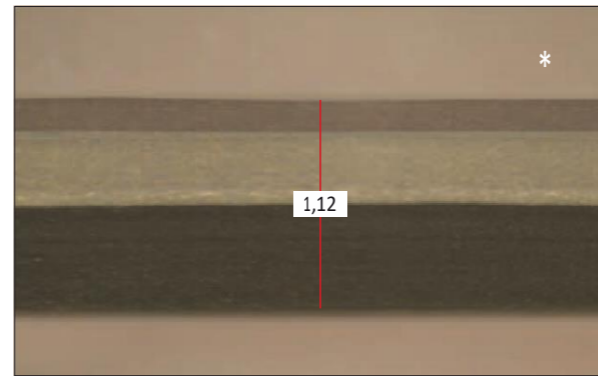
Рис. 4.3.8 Уменьшение толщины образца мембраны после испытаний в климатической камере после 10 условных лет. * толщина материала до испытания 1,23 мм
