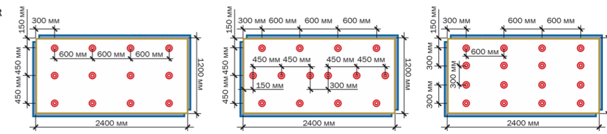
Рис. 2.3.3 Индукционная сварка
