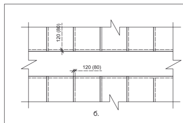
Рис. 5.4.2 Возможные варианты расположения рулонов мембраны
