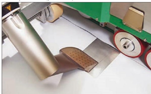
Рис. 5.2.6 Сварка с использованием металлической пластинки
