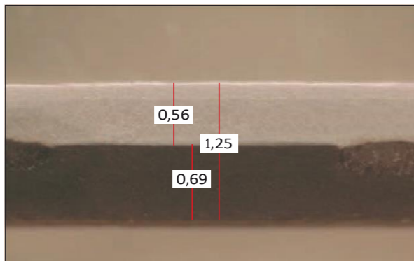
Рис. 4.3.6 Результаты испытаний кровельных мембран разной толщины
