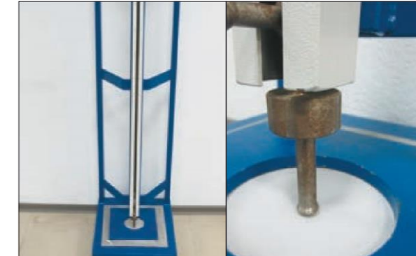
4.3.4 Общий вид установки для проведения испытания на ударную прочность
