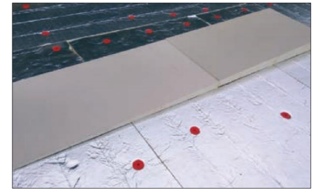
Рис. 3.3.12 Изображение PIR SLOPE с уклоном 1,7%
