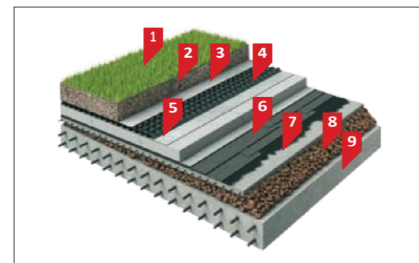
Рис. 2.7.4 Вид «зеленой» кровли
