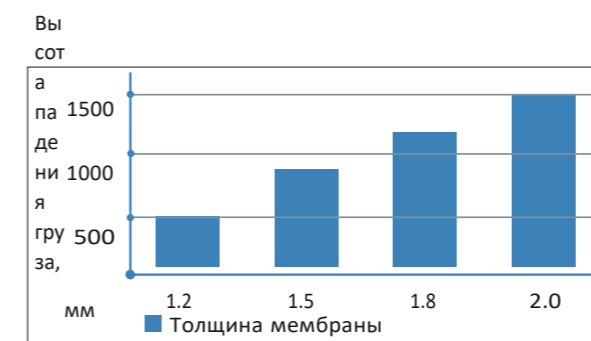
Рис. 4.3.2 Зависимость показателя ударной прочности от толщины мембраны. Образец мембраны толщиной 1,2 мм был прожжен насквозь. На кровле это может привести
