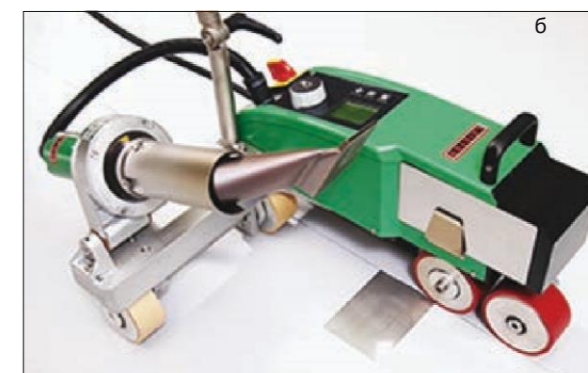
Рис. 4.8.13 Автоматическое сварочное оборудование
